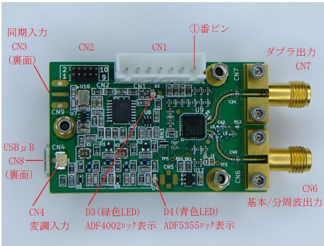
Fig.1 「びるる」PLL535L 外観
