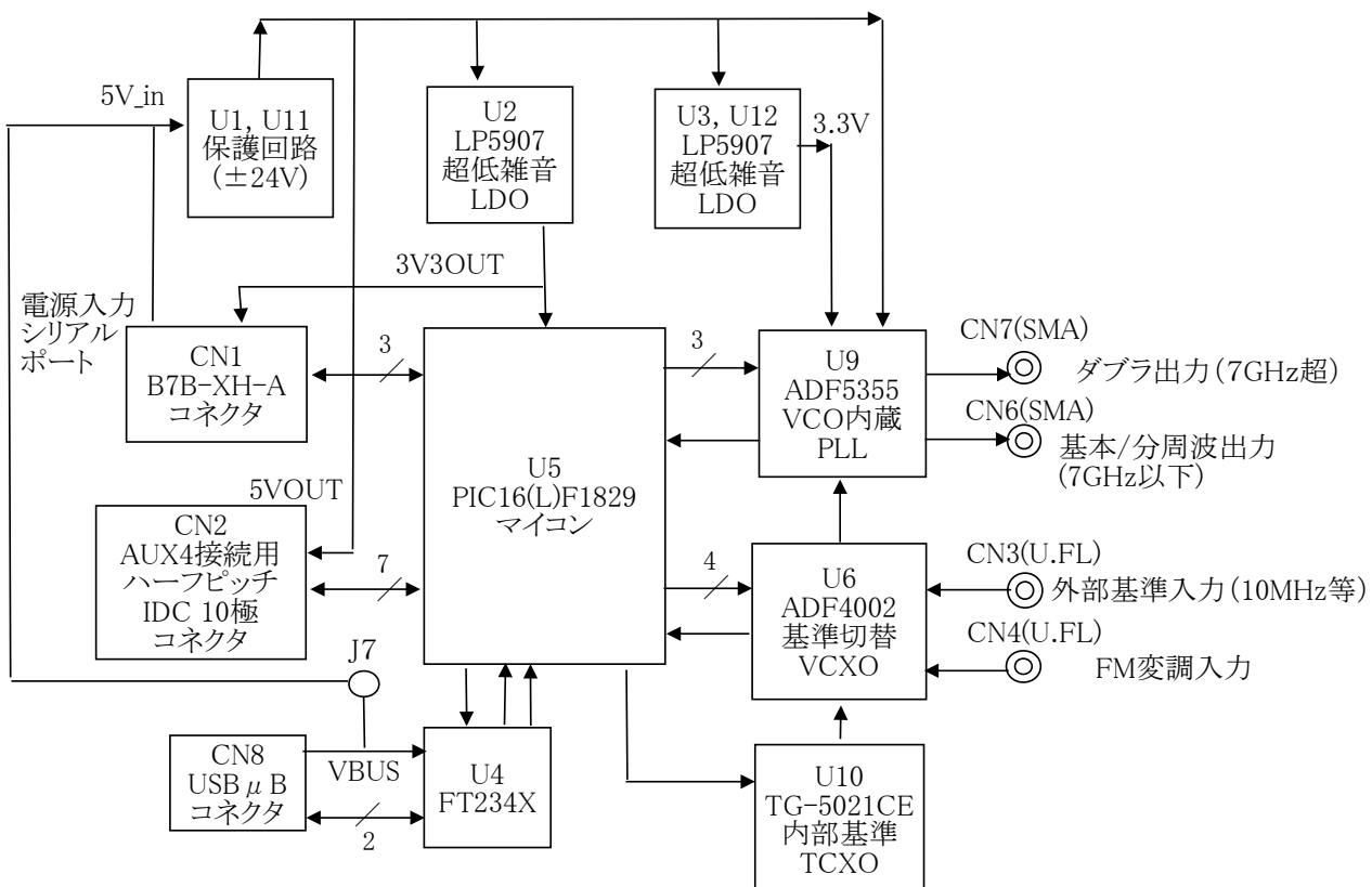
Fig.2 PLL535L ブロック図
