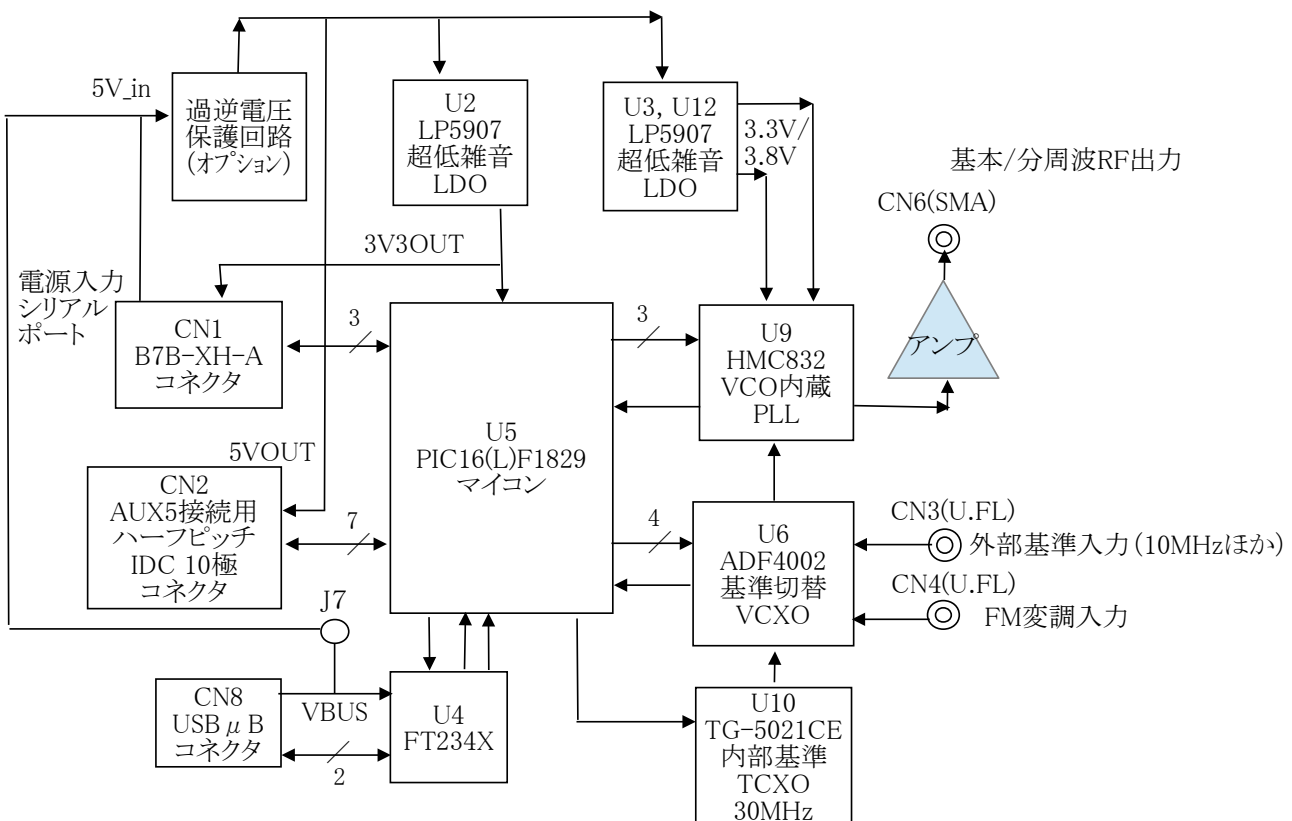
Fig.2 PLL832M ブロック図
