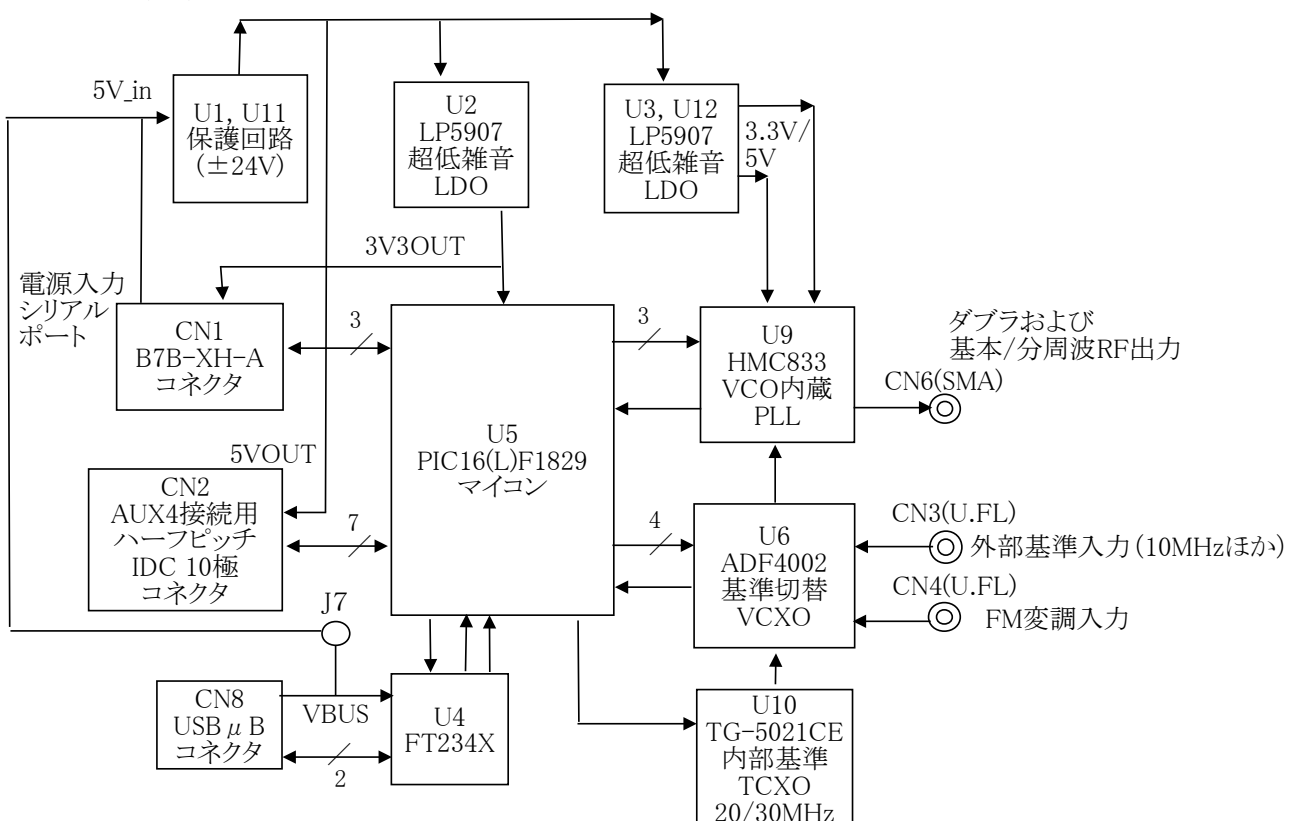
Fig.2 PLL833L ブロック図
