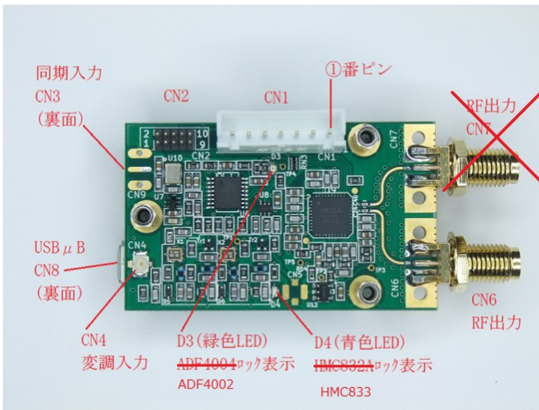
Fig.1 「びるる」PLL833L 外観
