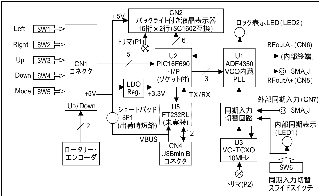
PLL352 ブロック図
